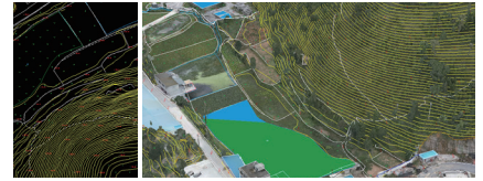
三维模型及线划图
