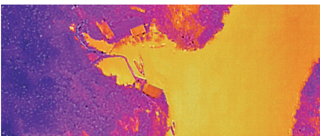
赤水河乌江排污口排查无人机监测热成像图
